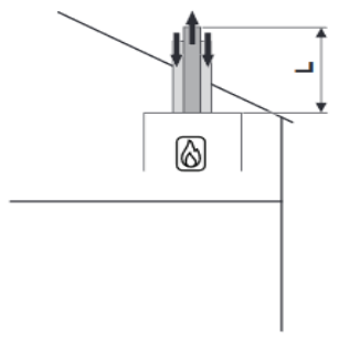
C33 Uygulama Örneği
