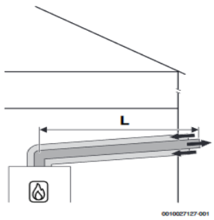
C13 Uygulama Örneği
