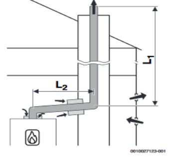
B Tipi Uygulama Örneği
