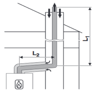
C93 Uygulama Örneği
